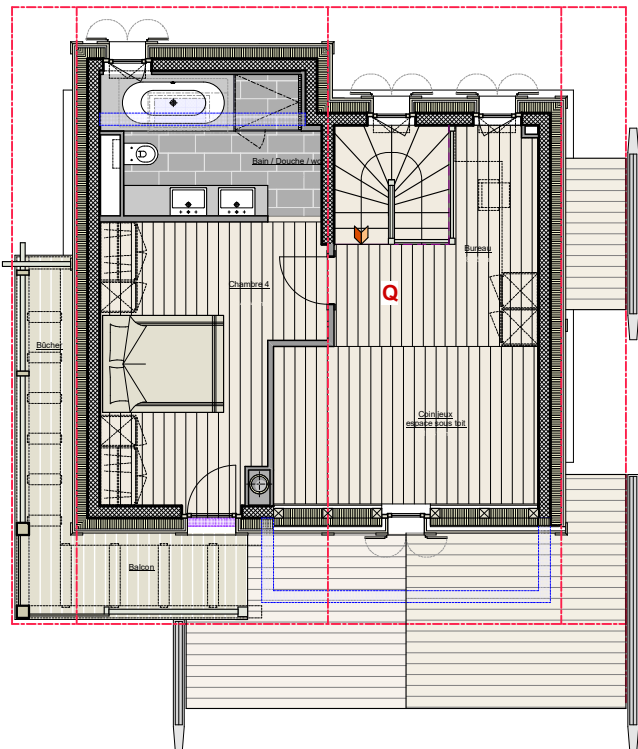
Chalet Q : Combles
