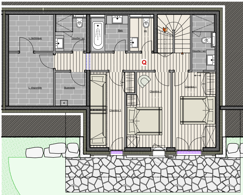
Chalet Q : Entresol
