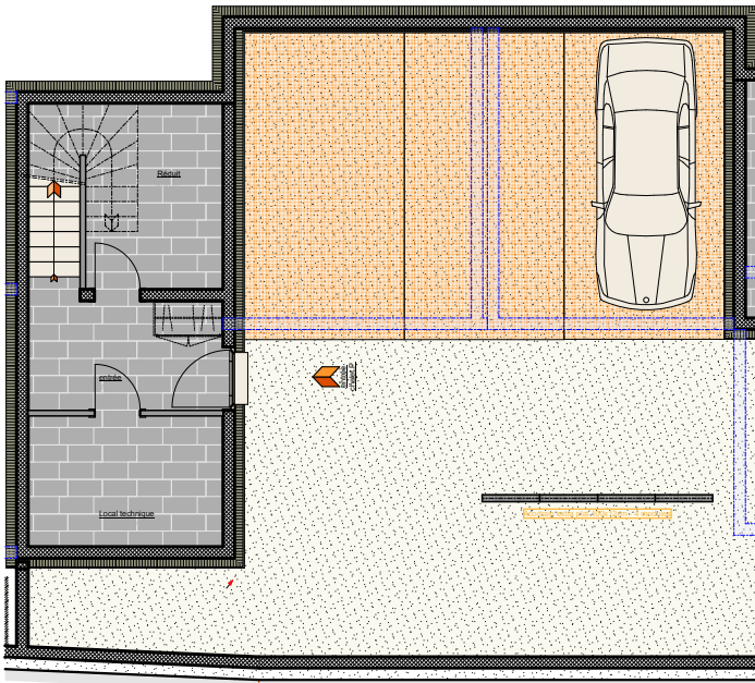
Chalet O : Garage
