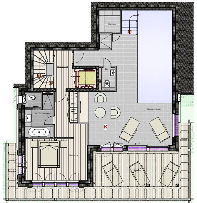
Chalet K : Entresol
