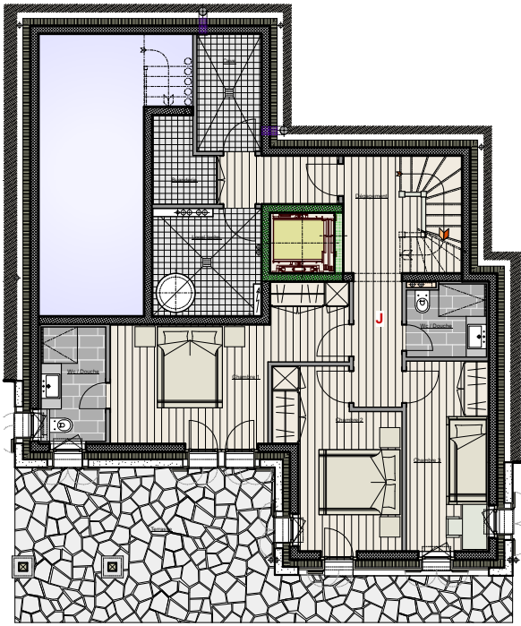
Chalet J : Sous-sol
