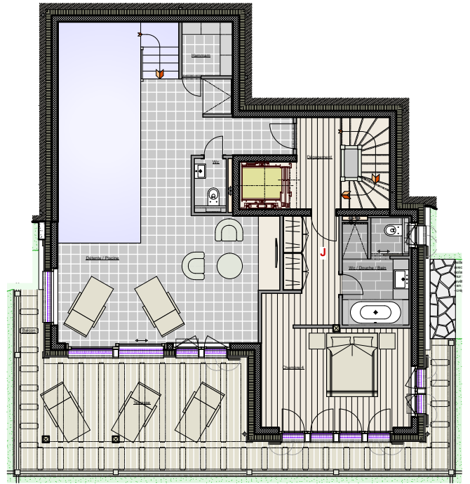
Chalet J : Entresol
