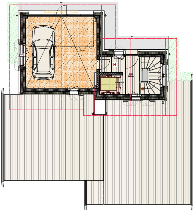
Chalet H : Combles
