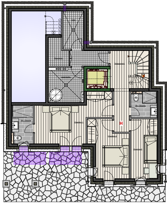
Chalet H : Sous-sol
