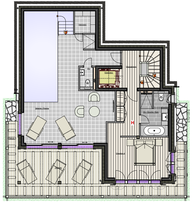
Chalet H : Entresol
