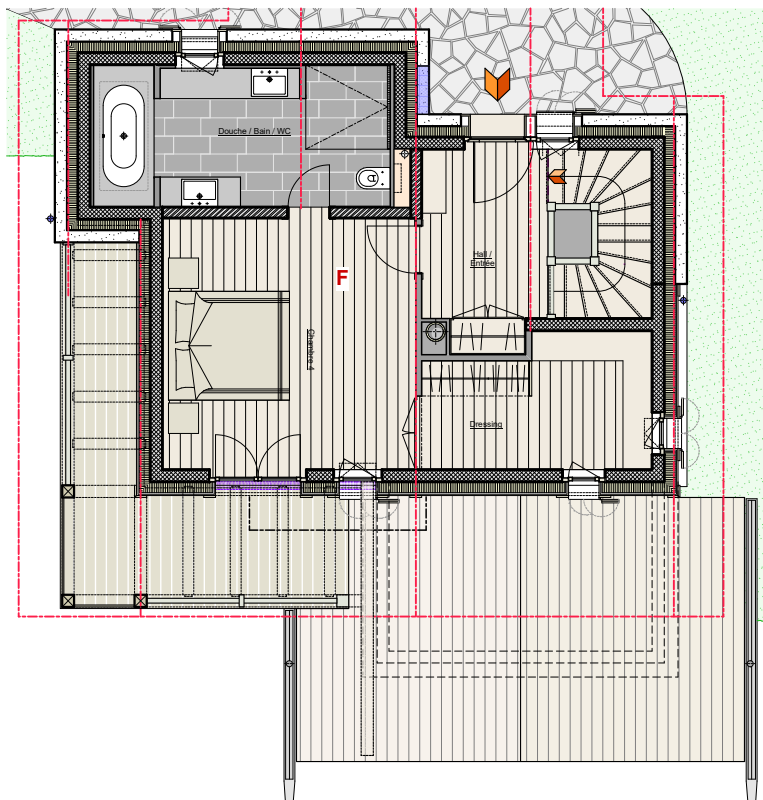
Chalet F : Combles
