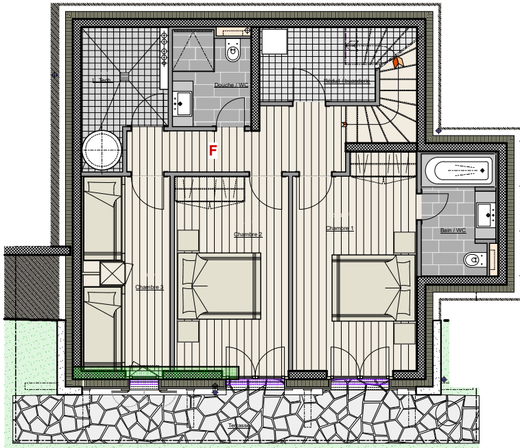
Chalet F : Entresol
