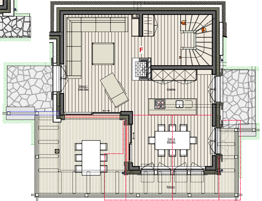
Chalet F : Etage
